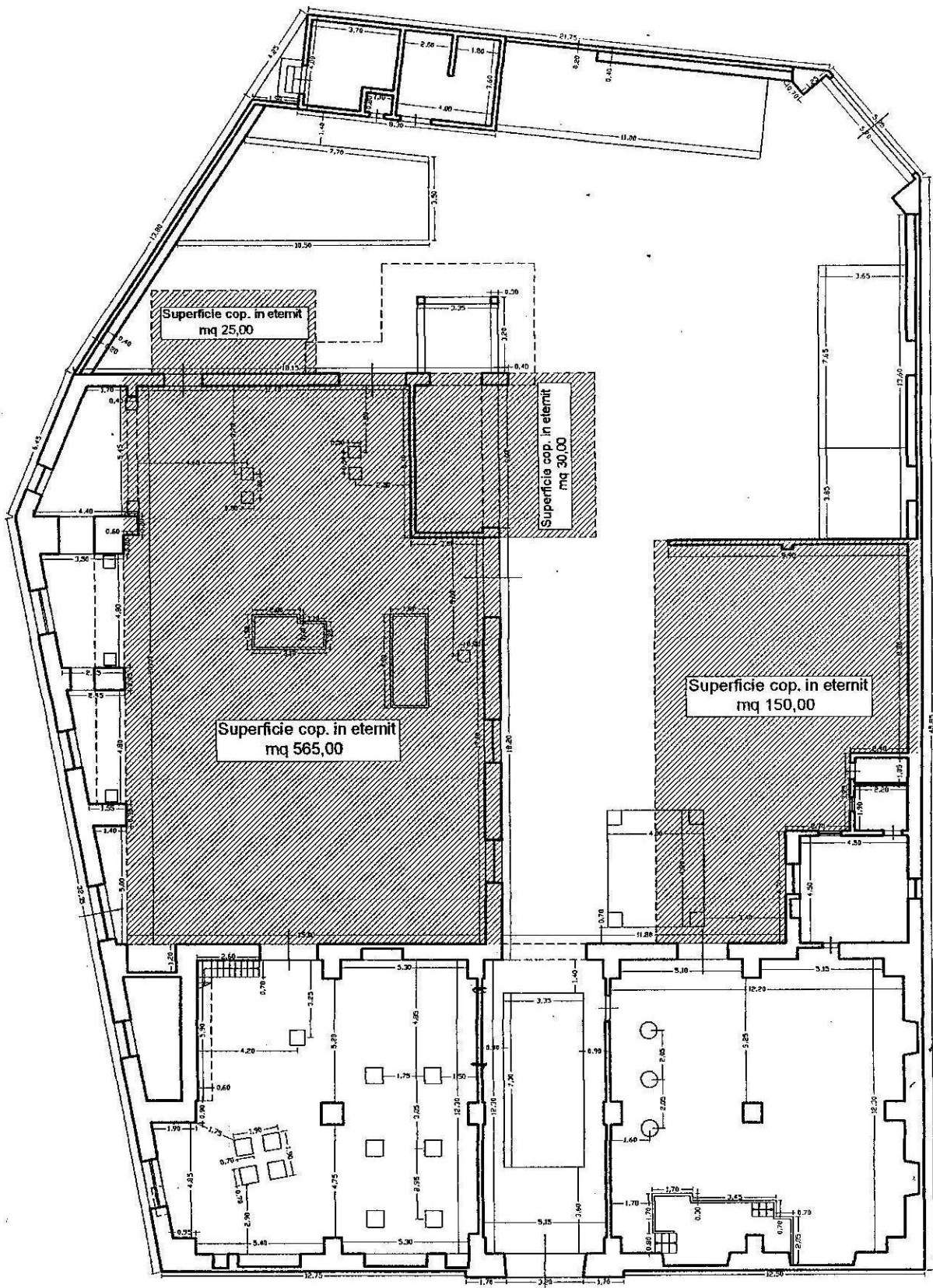
PLANIMETRIA COOP. SAN GIUSEPPE Rapp. 1:200
